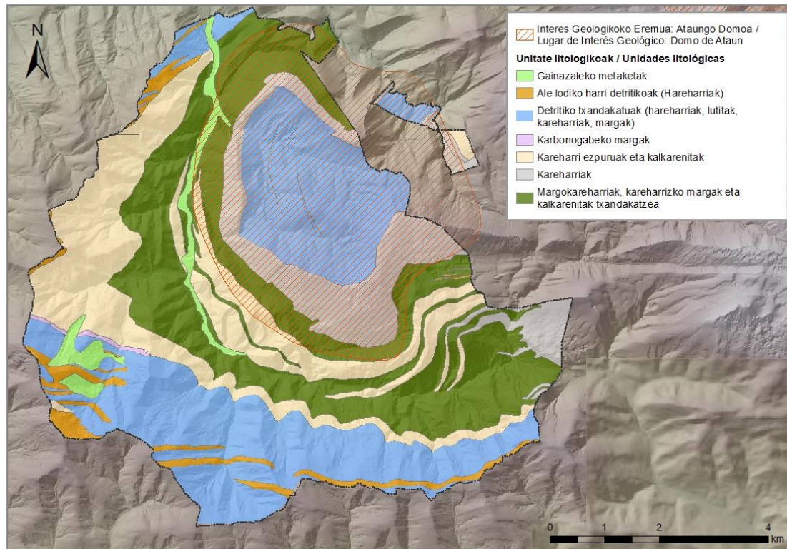
3. Irudia Ataungo unitate litologikoak
