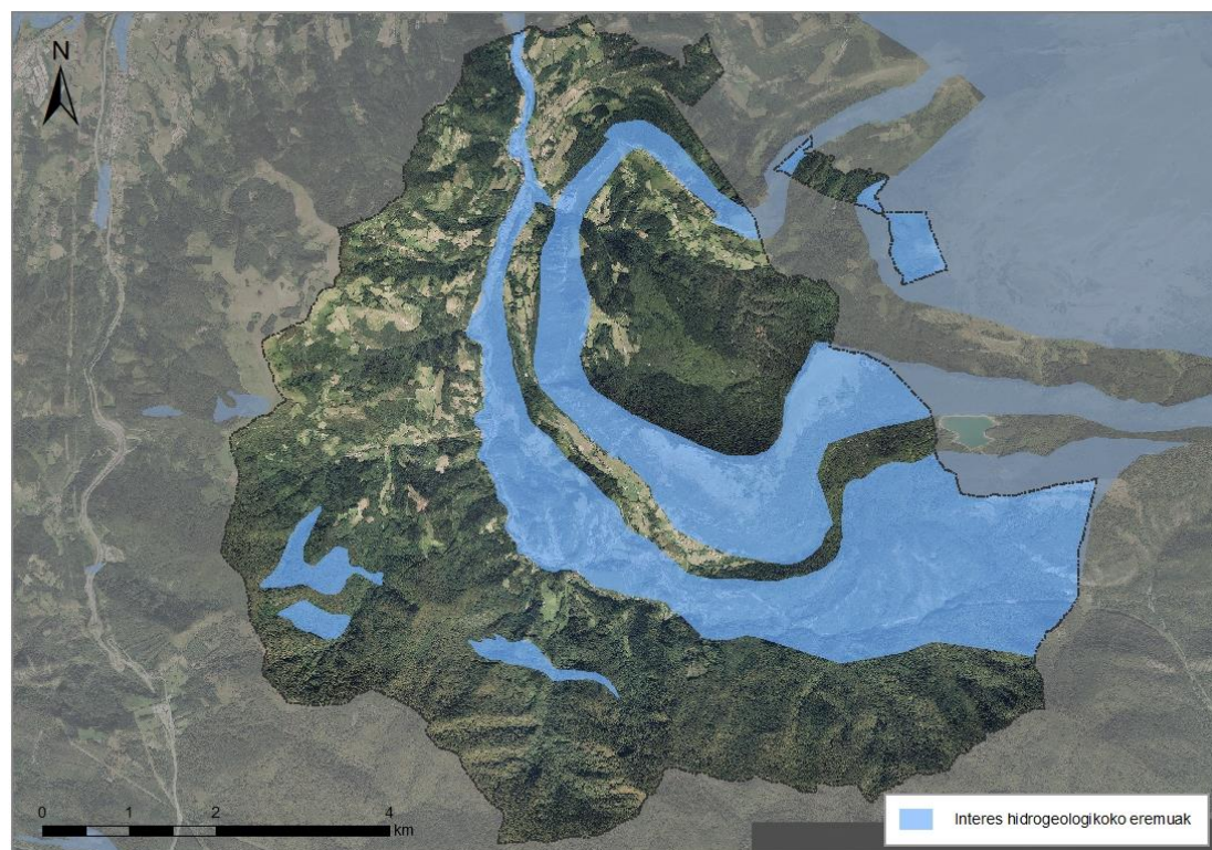
23. Irudia Interes hidrogeologikoko eremuak Ataungo udalerrian.
