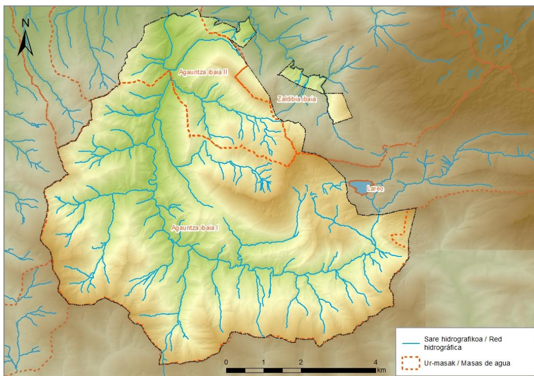
6. Irudia Sare hidrografikoa Ataungo udalerrian.
